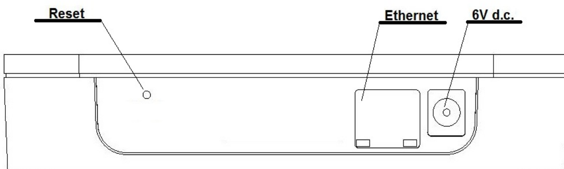
Rys.3. Widok części górnej rejestratora HT20
